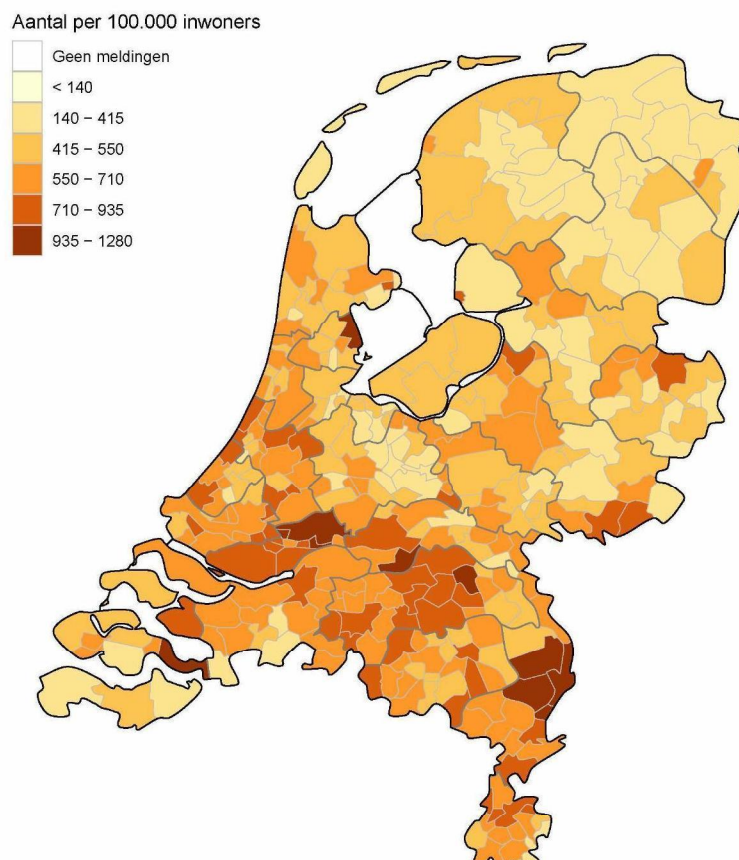
Figuur 11: Aantal aan de GGD'en gemelde personen met een positieve testuitslag voor SARS-CoV-2 per 100.000 inwoners per gemeente met GGD meldingsdatum van 2 april t/m 16 april 10:00 uur. De donkergrijze lijnen geven de grenzen van de GGD-regio's weer. De lichtgrijze lijnen geven de gemeentegrenzen weer.
