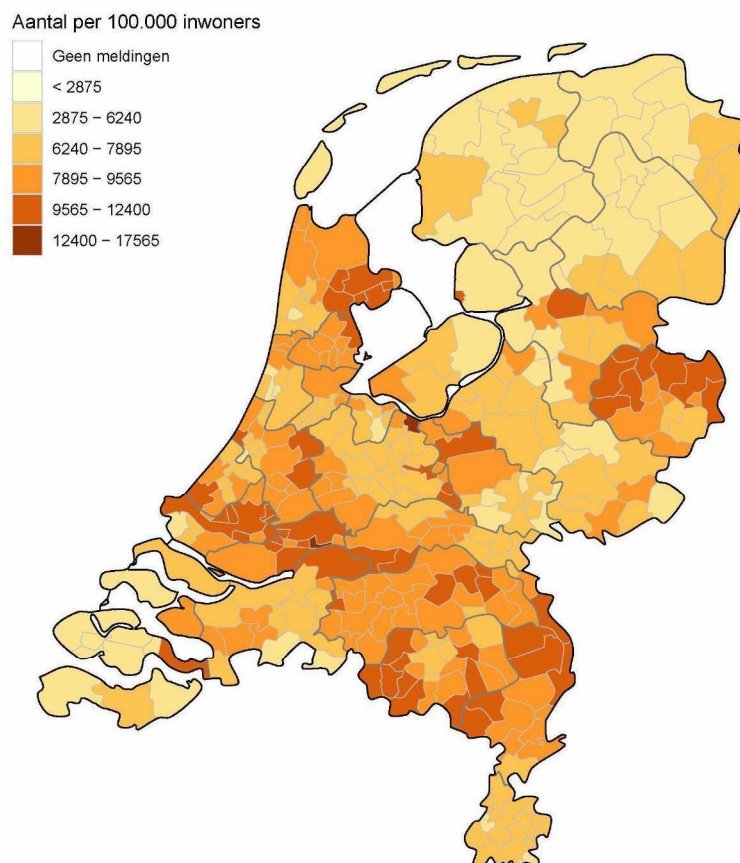
Figuur 46: Totaal aantal aan de GGD'en gemelde personen positief voor SARS-CoV-2 per 100.000 inwoners per gemeente t/m 16 april 10:00 uur. De donkergrijze lijnen geven de grenzen van de GGD-regio's weer. De lichtgrijze lijnen geven de gemeentegrenzen weer.
