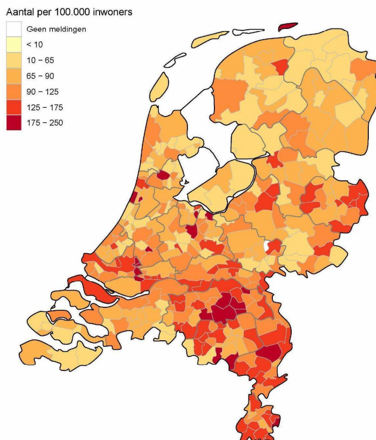
Figuur 47: Totaal aantal aan de GGD'en gemelde overleden personen positief voor SARS-CoV-2 per 100.000 inwoners per gemeente t/m 16 april 10:00 uur. Overlijden aan COVID-19 is niet meldingsplichtig en is daarom ondergerapporteerd. De donkergrijze lijnen geven de grenzen van de GGD-regio's weer. De lichtgrijze lijnen geven de gemeentegrenzen weer.
