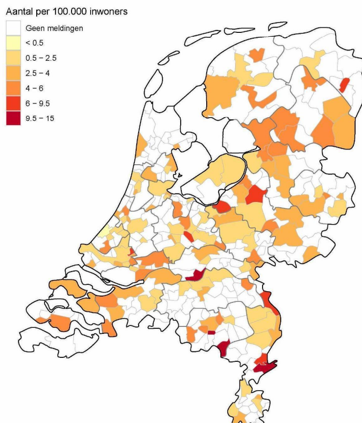
Figuur 12: Aantal aan de GGD'en gemelde overleden personen positief voor SARS-CoV-2 per 100.000 inwoners per gemeente met overlijdensdatum van 2 april t/m 16 april 10:00 uur. Overlijden aan COVID-19 is niet meldingsplichtig en is daarom ondergerapporteerd. De donkergrijze lijnen geven de grenzen van de GGD-regio's weer. De lichtgrijze lijnen geven gemeentegrenzen weer.
