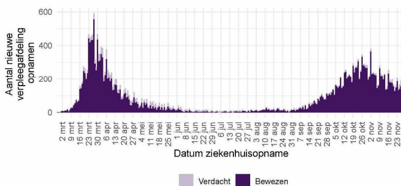
Figuur 37: Aantal nieuwe verdachte en bewezen COVID-19 patiënten per dag op Nederlandse 1 verpleegafdelingen.
