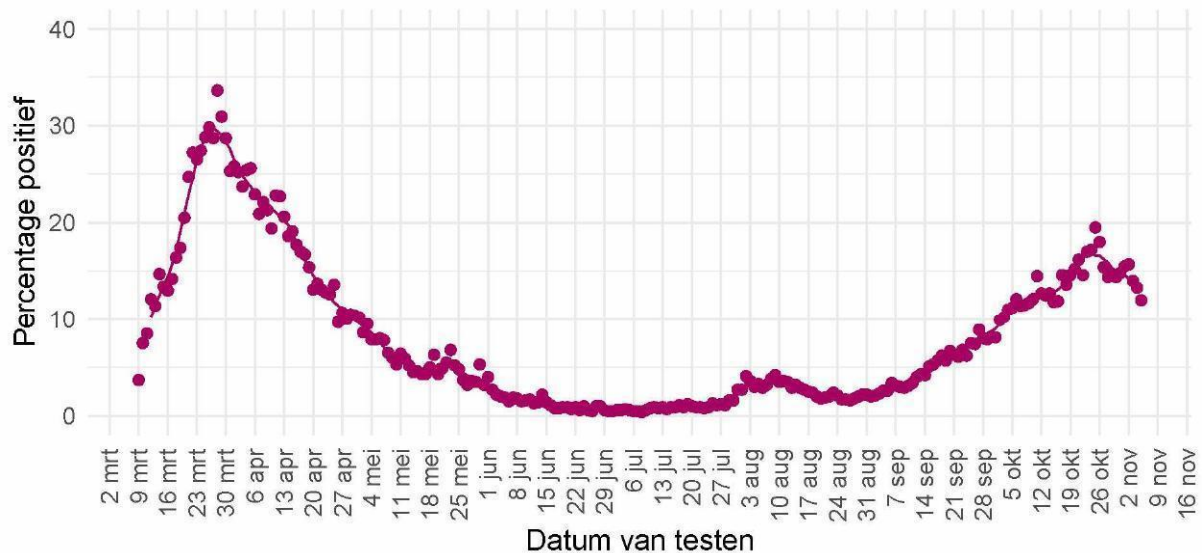
Figuur 27: Percentage van personen die getest zijn op SARS-CoV-2 waarbij de testuitslag positief was, gemeld door de virologische laboratoria. De stippen geven het percentage per dag aan; de lijn een 7-daags lopend gemiddelde.
