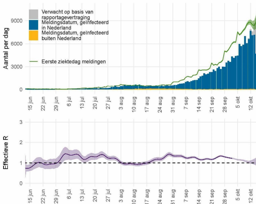
Figuur 26: Het effectief reproductiegetal R voor Nederland.
