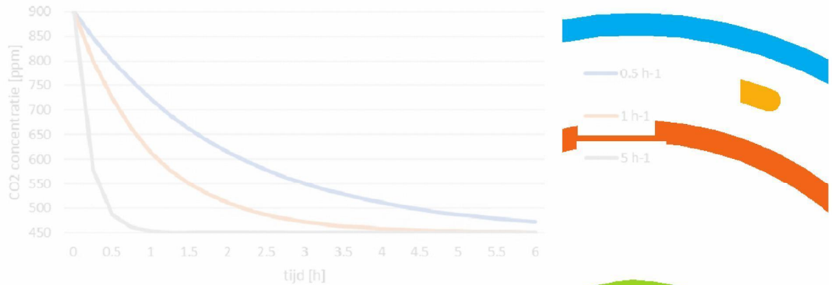
Afbeelding B9.1: Verloop van de CO 2 -concentratie bij verschillende waarden voor het ventilatievoud ( C_0 = 450 ppm, C_{\text{eind}} = 900 ppm)
